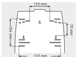
Assemble des trous de fixation
