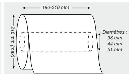
Dimensions des bobines compatibles
